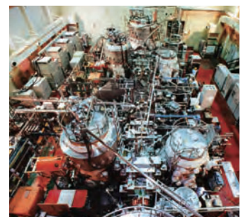
Fig: プラズマ実験装置ガンマ10
